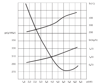
Diagramma consumo e potenza
